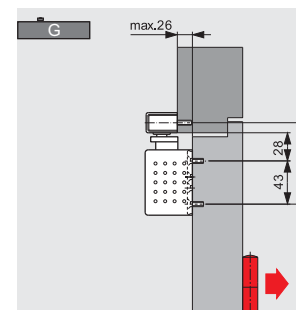
Montaje en retranqueo en el lado de las bisagras
